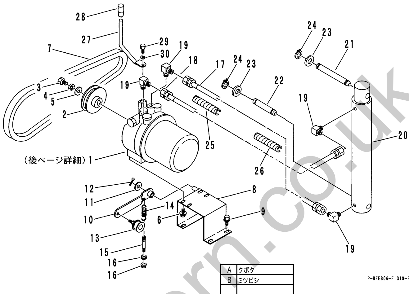
FIG 19 ユアツソウチ (ダンプ) HYDRAULIC SYSTEM (DUMP)
